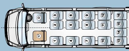
16+D / 17+D (3700 WB)
